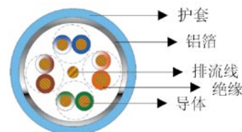
Cat5e F/UTP
