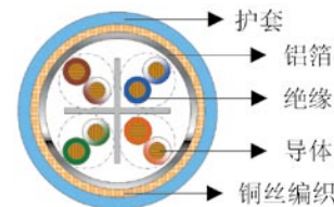
Cat5e SF/UTP
