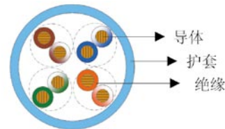
Cat5e U/UTP
